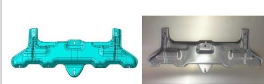
Haltewinkel - Aluminium
