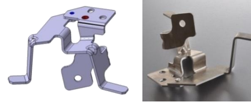
Armaturentafelhalter - Aluminium
